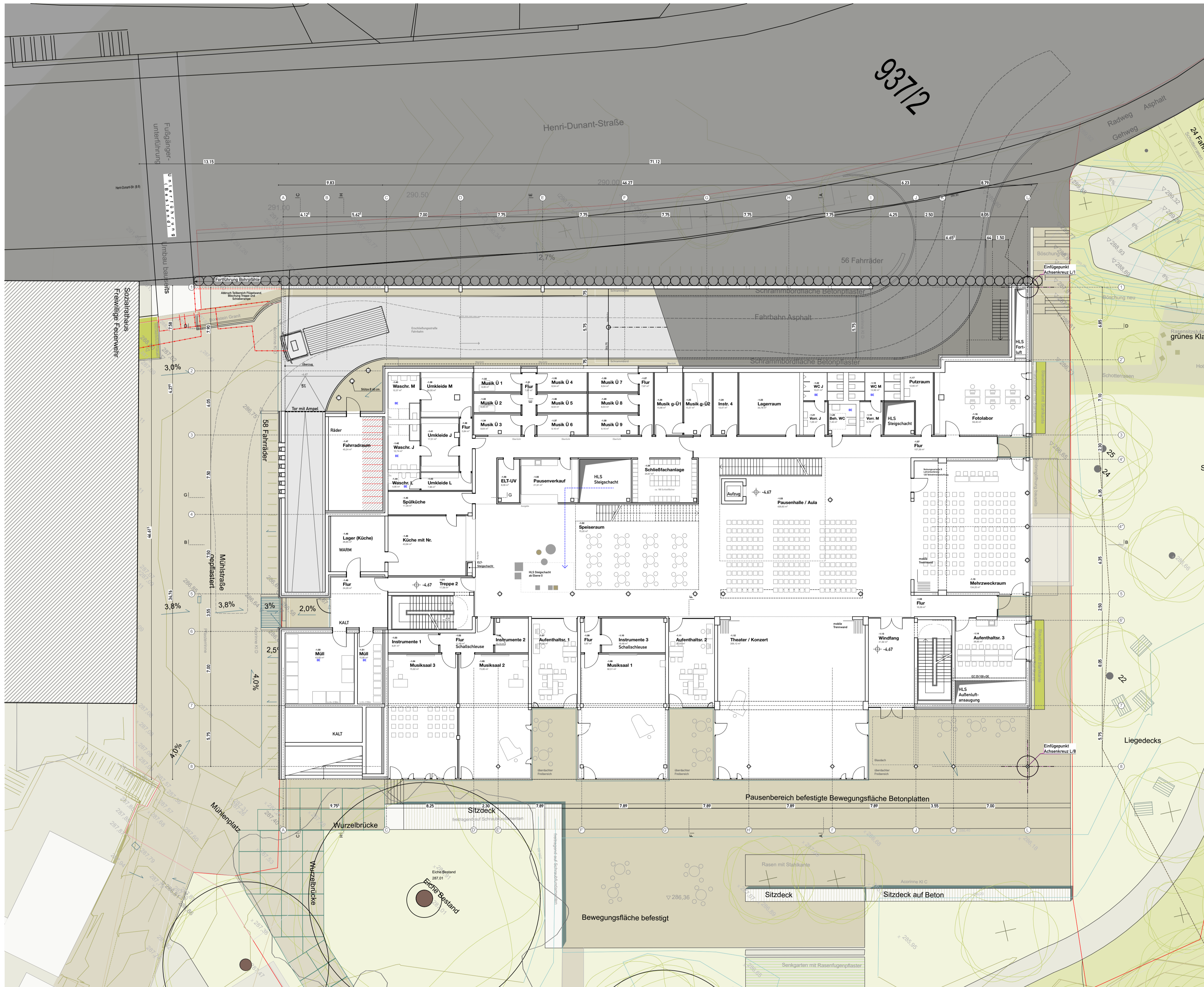
GRUNDRISS Ebene -1 1:200
