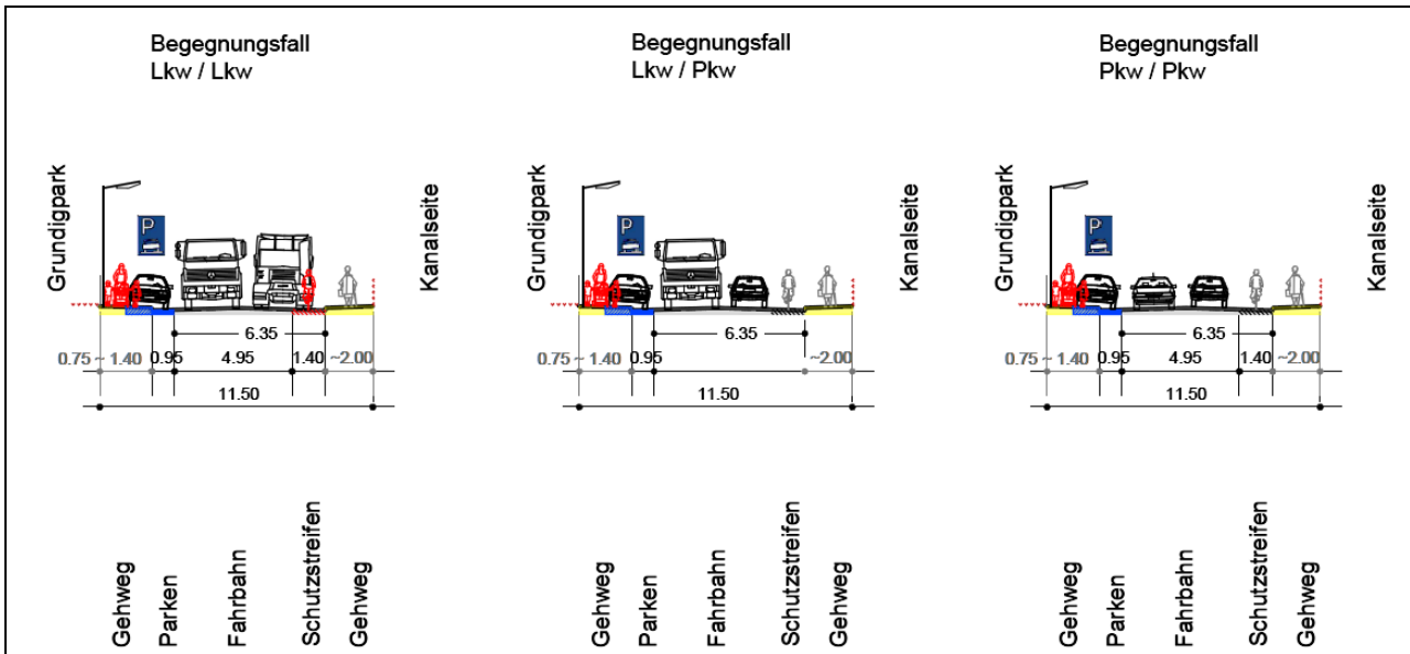
Abb. 4: Querschnittsgestaltung der Straße Am Europakanal (halbseitiges Gehwegparken, Auflösung Schutzstreifen)
