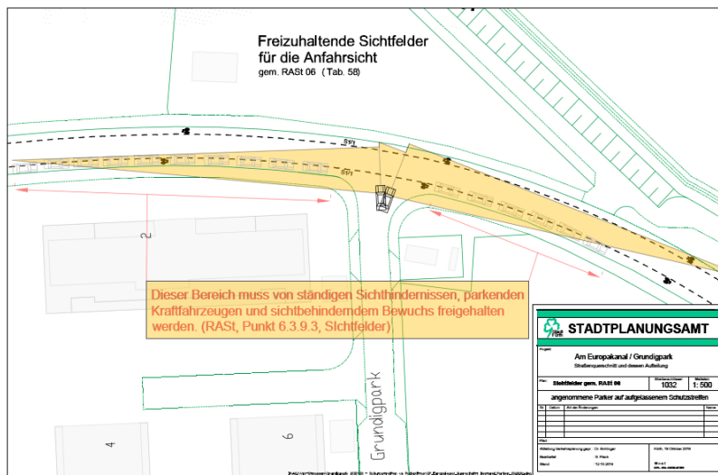
Abb. 5: Sichtfelder im Einmündungsbereich Grundigpark / Am Europakanal
