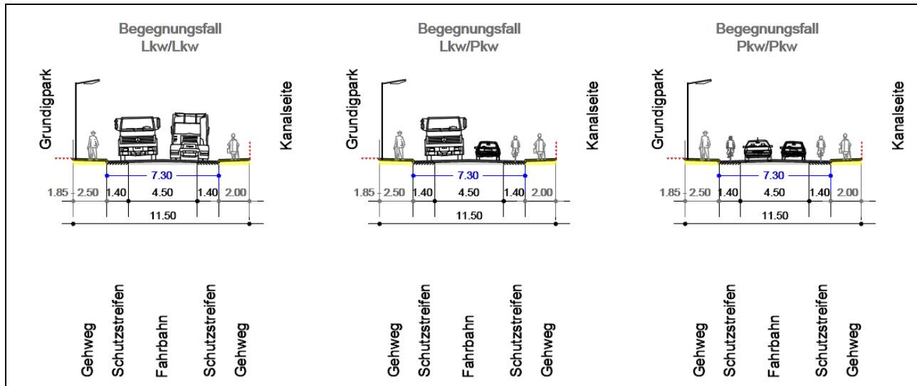
Abb. 2: Querschnittsgestaltung der Straße Am Europakanal (Bestand)
