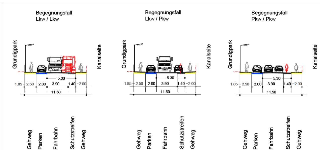
Abb. 3: Querschnittsgestaltung der Straße Am Europakanal (Parken auf der Fahrbahn, Auflösung Schutzstreifen)
