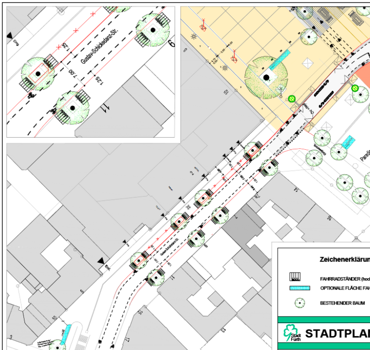
Abb. 1: Ausschnitt Lageplan
