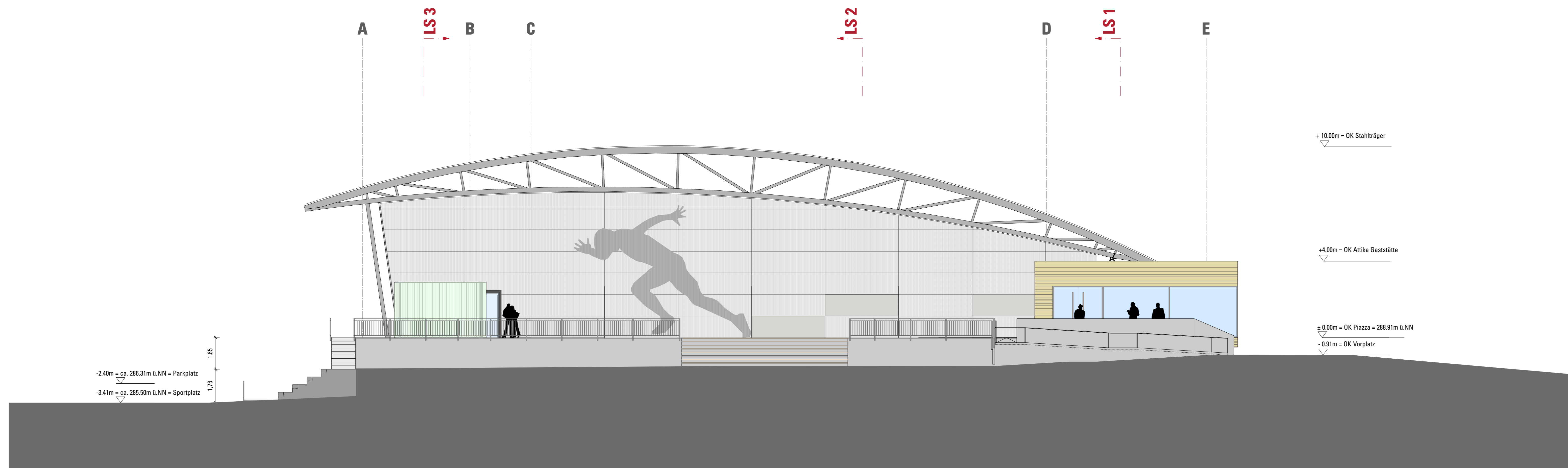
Ansicht AR-BA-AN01-210 Norden 1-100
