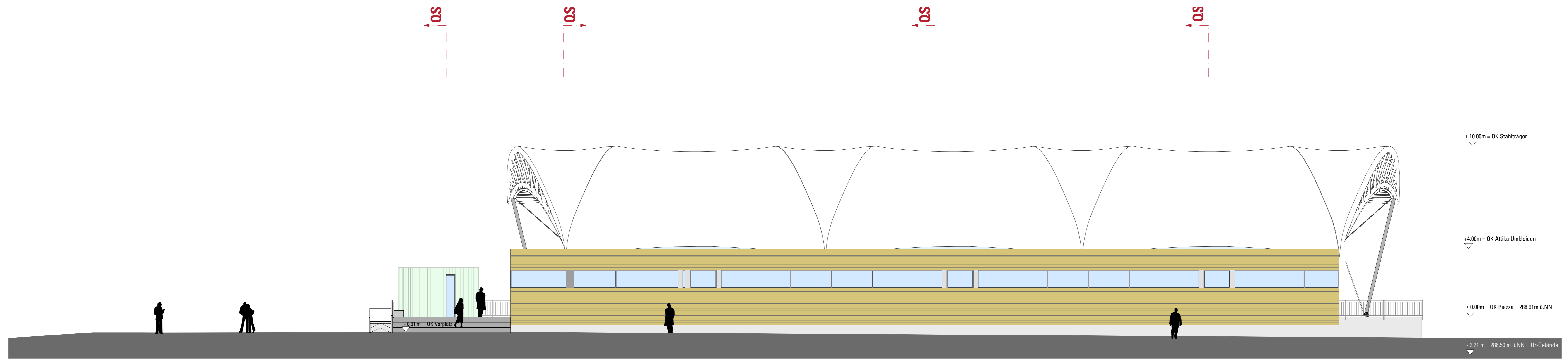
Ansicht AR-BA-AN03-230 Westen 1-100
