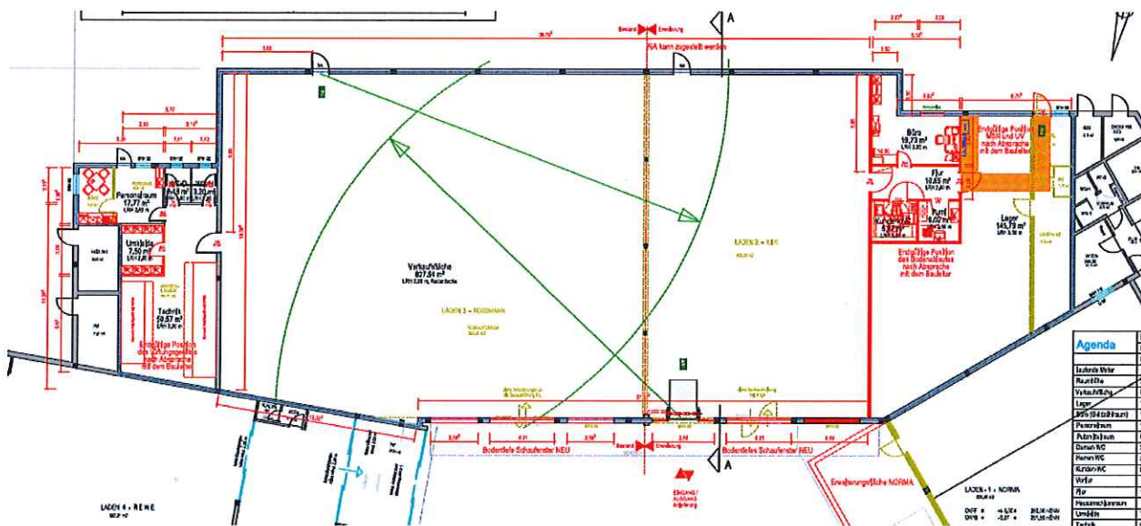
Anlage 4: Erweiterung Rossmann auf KiK Fläche
