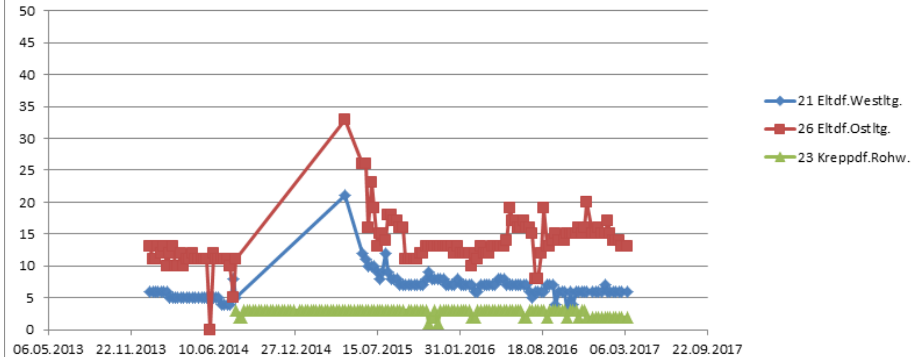
Nitratkonzentrationen der Rohwassersammelleitungen der Wasserwerke des ZV Eltersdorfer Gruppe in mg/l
