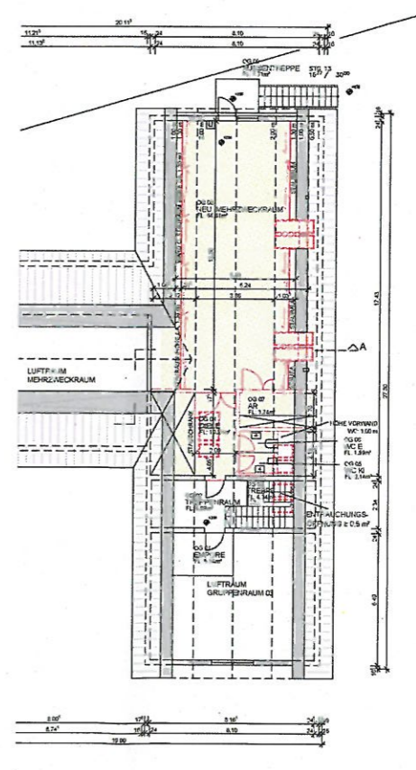
GRUNDRISS DACHGESCHOSS
