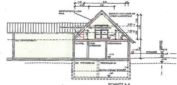
SCHNITT A-A
