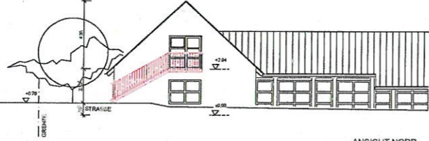
ANSICHT NORD
