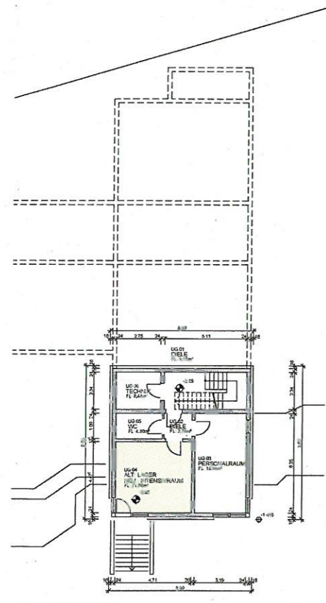
GRUNDRISS UNTERGESCHOSS
