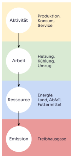
Abbildung 1: CO 2 -Wirkungskette
