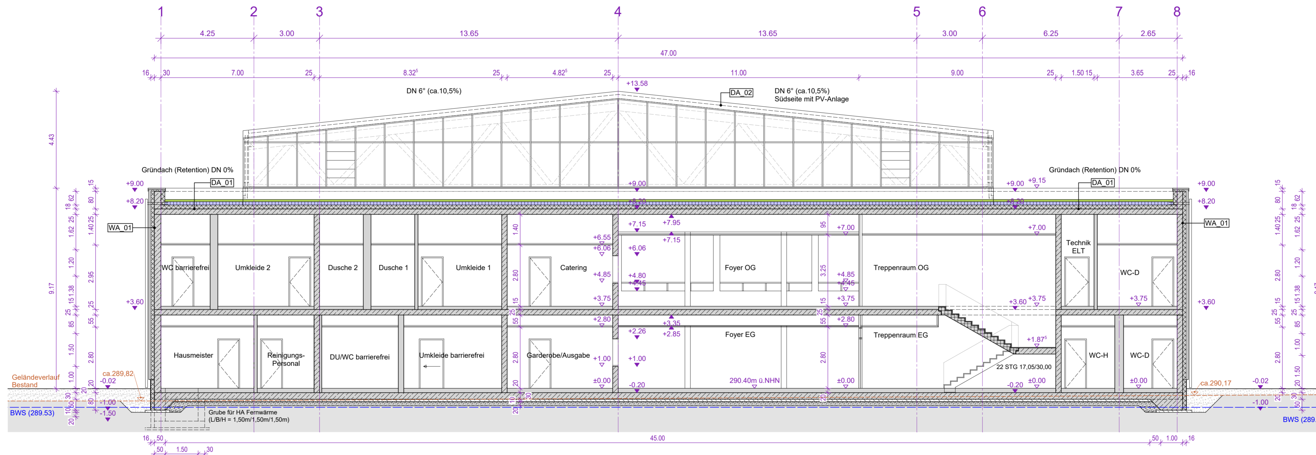
SN3 - Schnitt Foyer/Treppenraum
