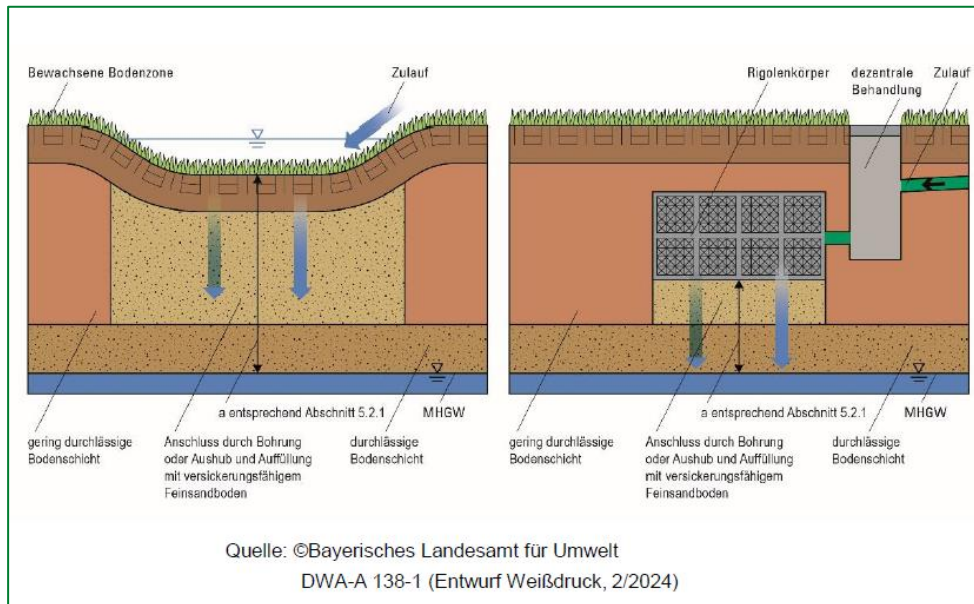
Abbildung 4: Aufbau Versickerungsmulde und Rigolen mit Bodenaustausch nach DWA-A 138-1 (Landesamt für Umwelt, 2024).
