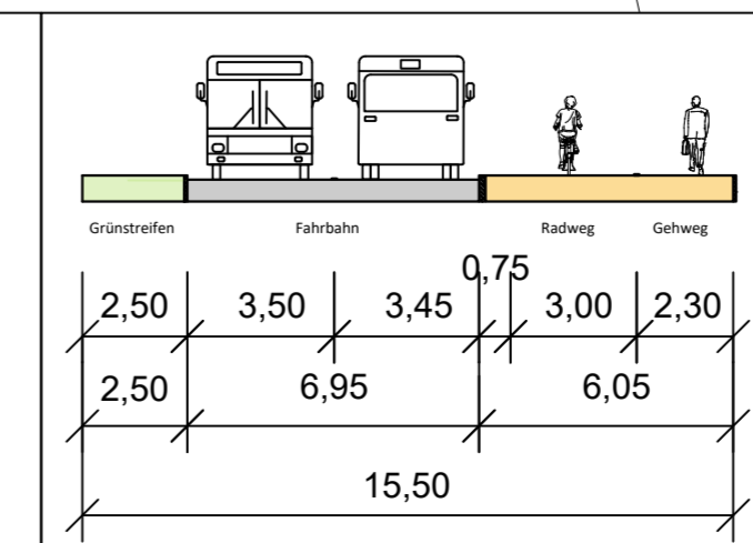
Regelquerschnitt B - B
