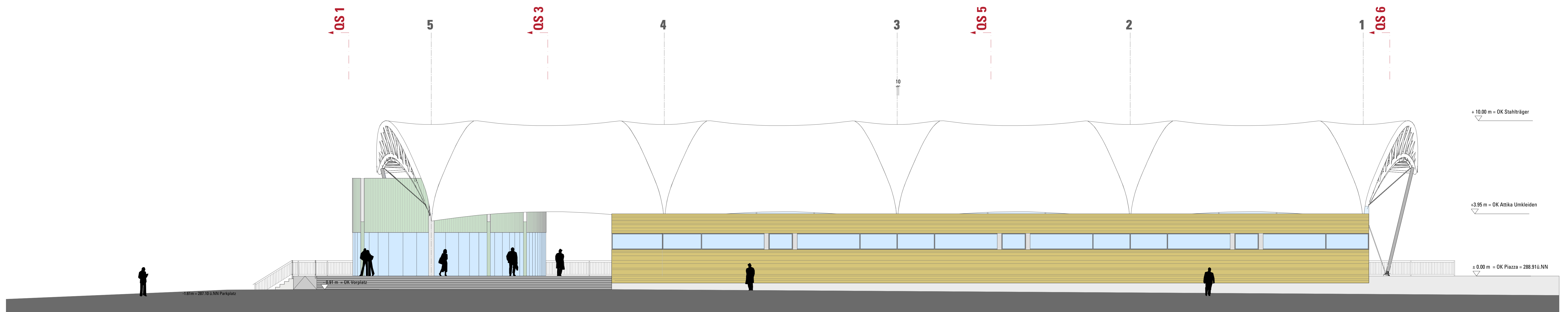
Ansicht AR-BA-AN03-230 Westen 1-100
